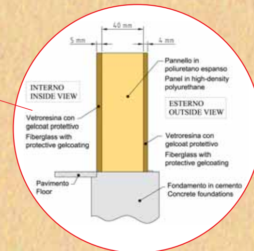
Dettaglio interno di un modulo Fiberbox 150 Inside detail view of a module Fiberbox 150 Vue d'un détail intérieur d'un module Fiberbox 150 Detailbild der Innenausstattung bei einem Modul Fiberbox 150
