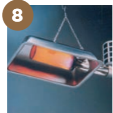
8 Cappe riscaldanti e generatori di aria calda per i pulcini. Heating systems like gas brooders particularly suitable for chicks during first days and air-blowers powered both by gas or diesel. Capes chauffantes et générateurs d'aire chaude pour les poussins. Heizhauben und Warmluftverzeuger für Küken. Системы обогрева, такие как брудеры с газовым обогревом, особенно подходят цыплятам в первые дни жизни, и воздуходувки
